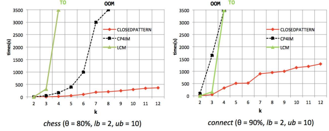
FIGURE 1 – k motifs avec CLOSEDPATTERN, CP4IM, LCM
