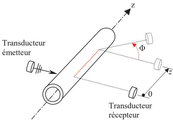
Figure 3 : configuration (2) bistatique expérimentale. Le transducteur émetteur est fixe ; le transducteur récepteur, repéré par l'angle \Phi , tourne dans un plan azimutal comprenant le transducteur émetteur et l'axe de l'objet.
